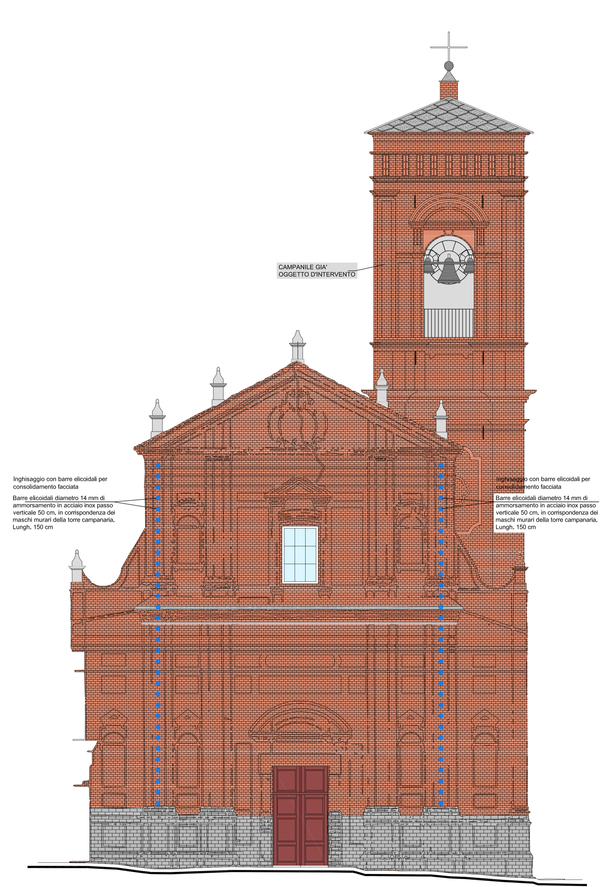
PROSPETTO FACCIATA PRINCIPALE SCALA 1:100
